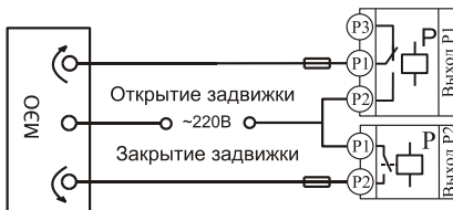
Подключение электрозадвижки
