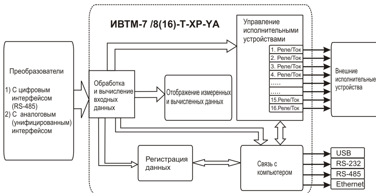
Рисунок 3.14 Функционирование прибора
