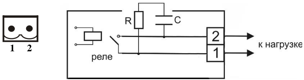
Рисунок 3.12 Подключение нагрузки к выходу управления
