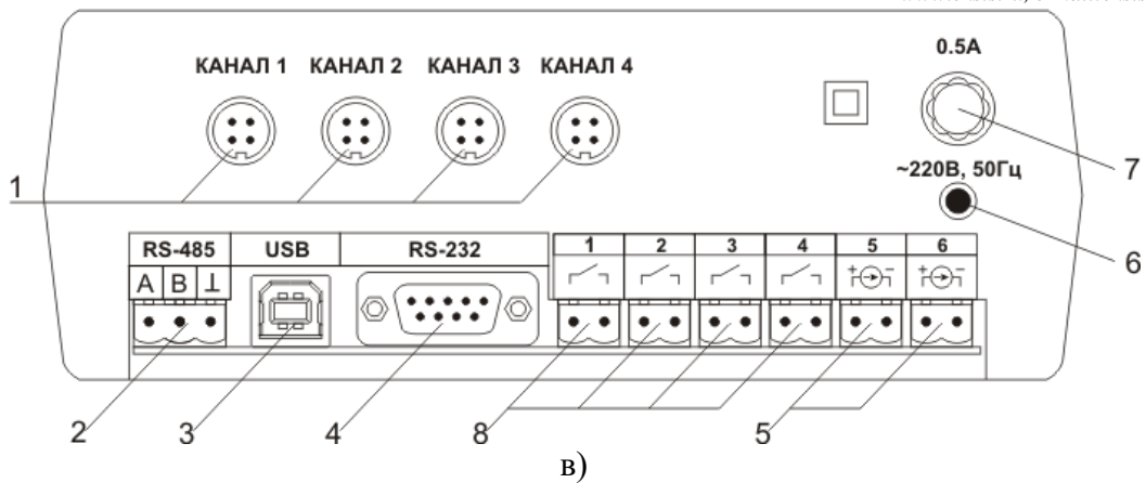
Рисунок 3.3 Вид задних панелей приборов ИВТМ-7 /Х-Т-4Р-2А:
