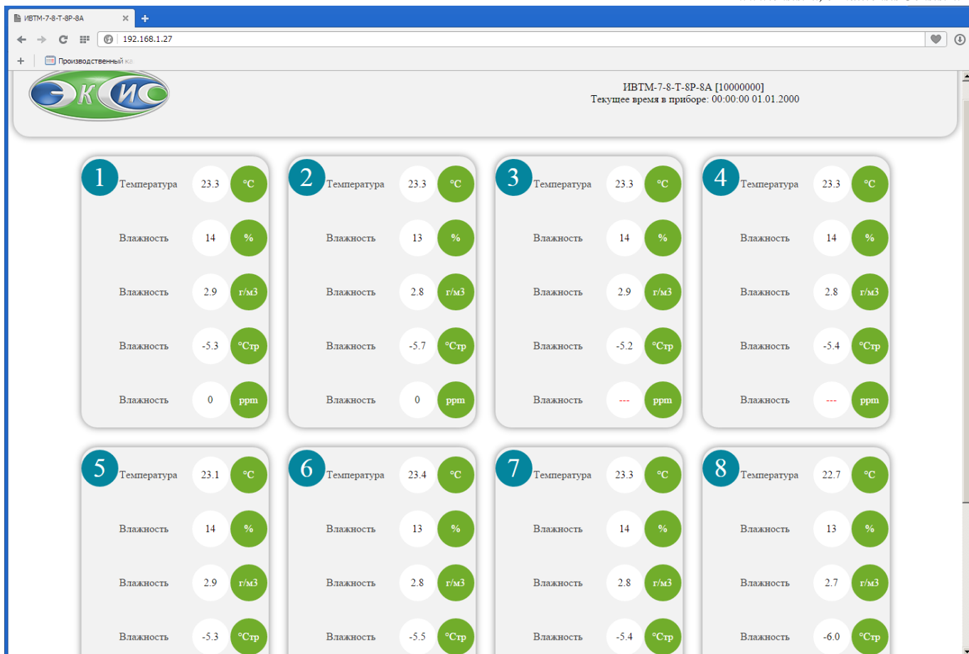
Рисунок 6.27 Web-интерфейс прибора ИВТМ-7 /8-T-УР-ZA.
