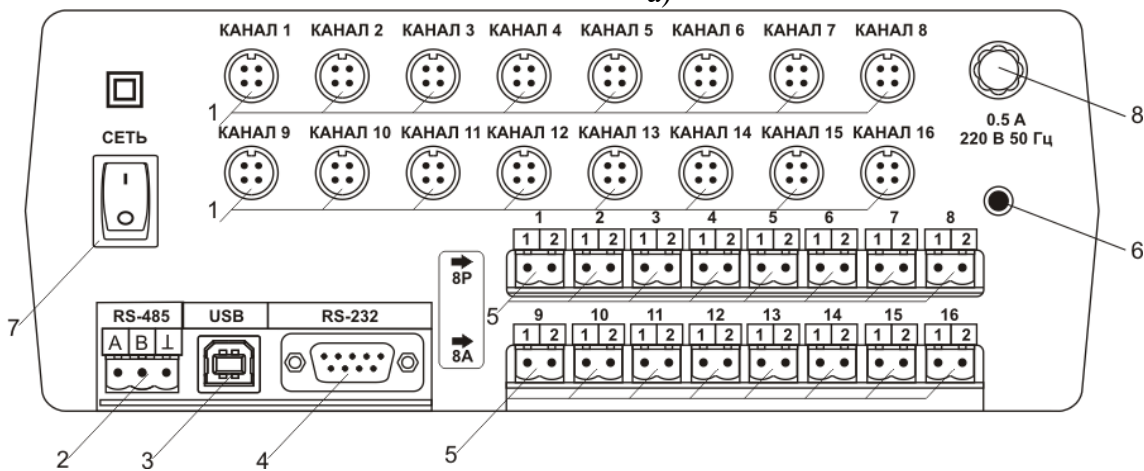
Рисунок 3.6 Вид задних панелей приборов ИВТМ-7 /8(16)-Т-8Р-8А (5”):
